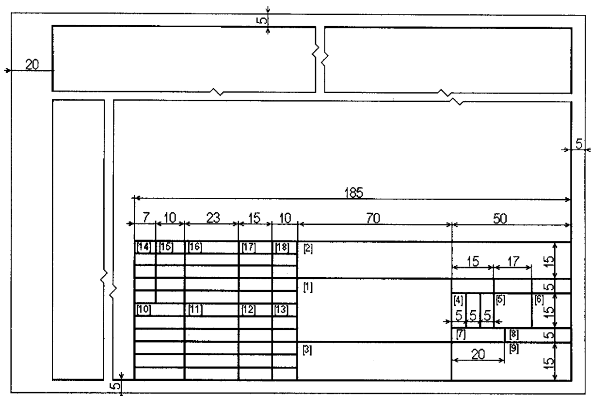
Рисунок К.1 – Правила оформления основной надписи на формате (поле чертежа)
